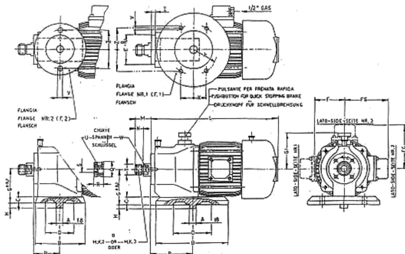
DIMENSIONI - DIMENSIONS TABLE - MAßTABELLE
